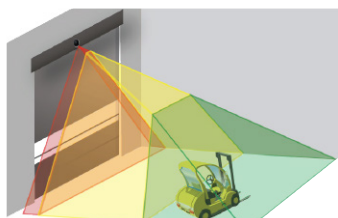
La zone verte agit comme un détecteur de mouvement. La zone jaune agit comme un détecteur de présence.
